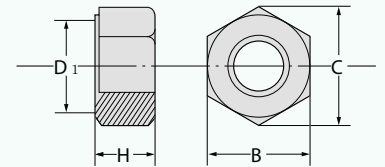
NUT
